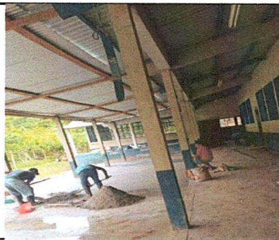
Foto 6: Fundición de piso en el corredor.
